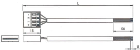
CBL SET GL5 (P/N: 804150) GL5 cable connector
