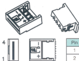
CON GL5 (P/N: 807086) GL5 connector
